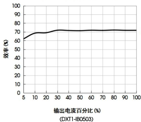
效率Vs输出负载 (Vin=12V)
