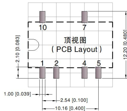
引脚方式
